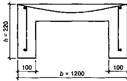
Рисунок 1 – Сечение плиты
