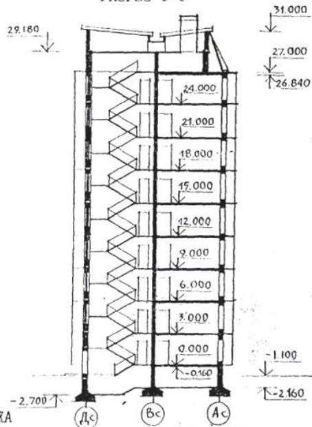
РАЗРЕЗ I-I
