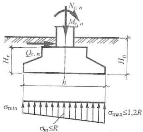
Рисунок 2 – Внецентренно нагруженный фундамент
