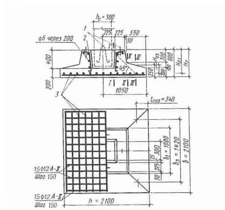
Рисунок 1 - Центральна-нагруженный фундамент
