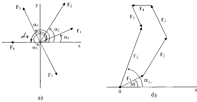
Рисунок 1 – Многоугольник сил
