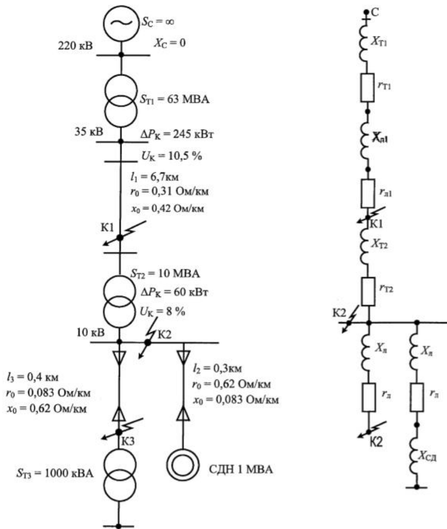
Рисунок 1 – Исходная схема (а) и схема замещения (б)
