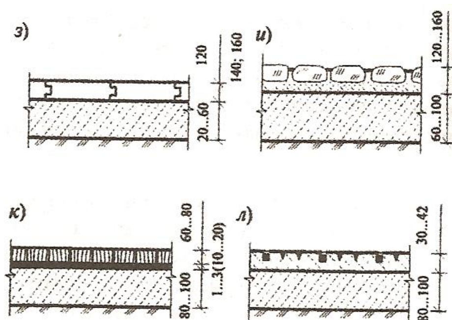
Рисунок 66 – Полы
