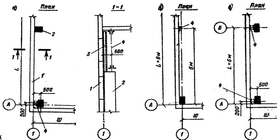
здания, L=9\text{м} , стена прислонена к колоннам каркаса; в) то же, L=6\text{м} , колонны каркаса отодвинуты от разбивочной оси; t – панельная стена; 2 – колонна фахверка; 3 – верхняя (стальная) часть колонны; 4 – стальная приколонная стойка фахверка
