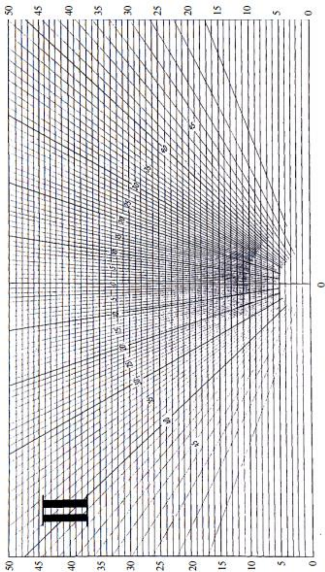
Рис. 8. График П. А. М. Данилова для подсчета n_2 и n_2'
