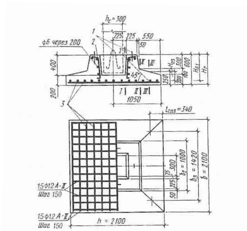
Рисунок 1 - Централь-но-нагруженный фундамент
