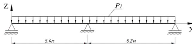
Рисунок 12 - Схема загрузки 2
