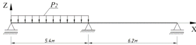
Рисунок 13 - Схема загрузки 3
