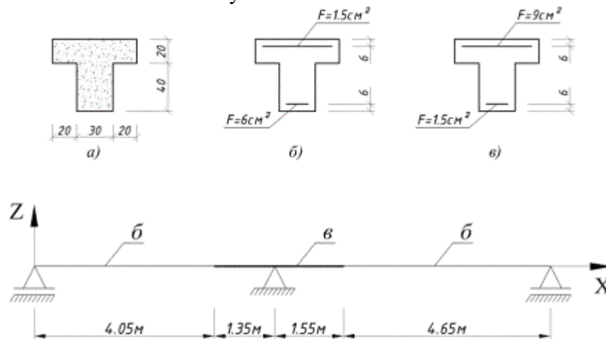
Рисунок 9 – Схема балки
