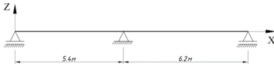
Рисунок 9 – Схема балки
