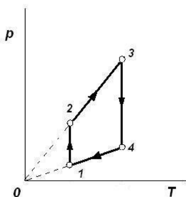
Рис. 1. График изопроцессов в координатах РТ
