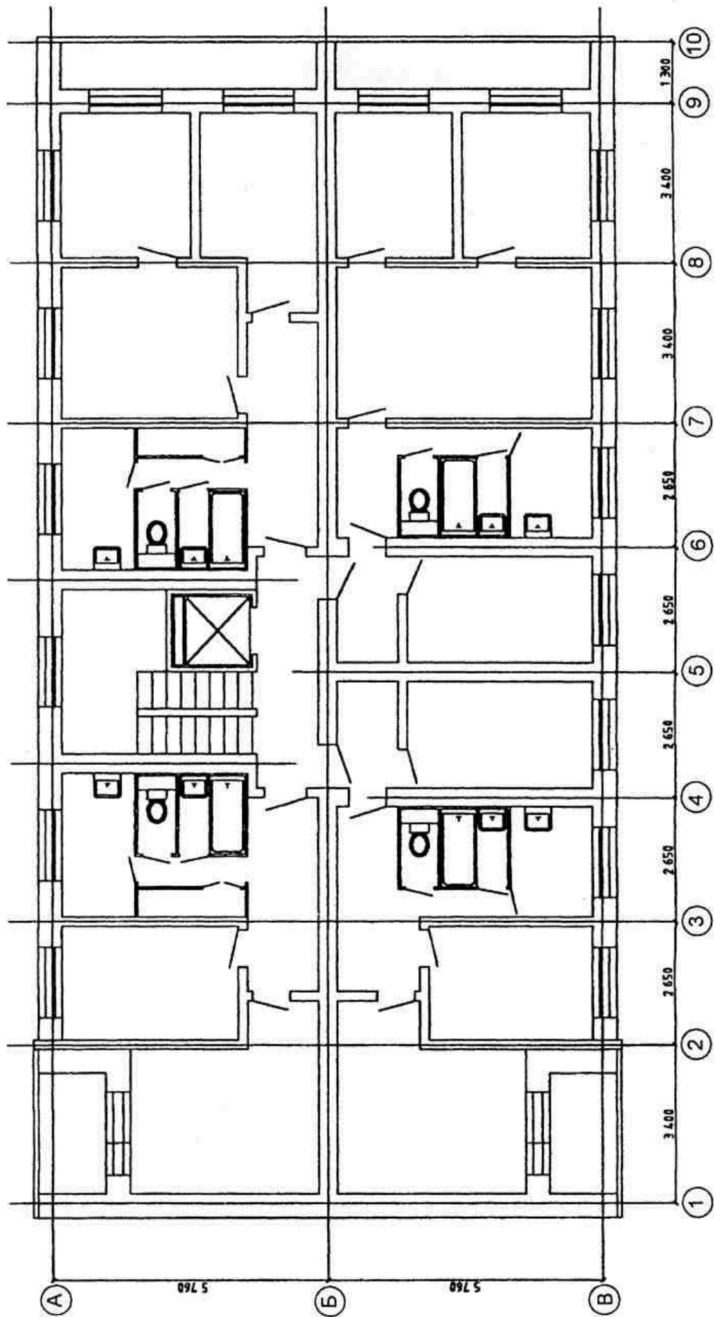
ПЛАН ТИПОВОГО ЭТАЖА М 1:100
