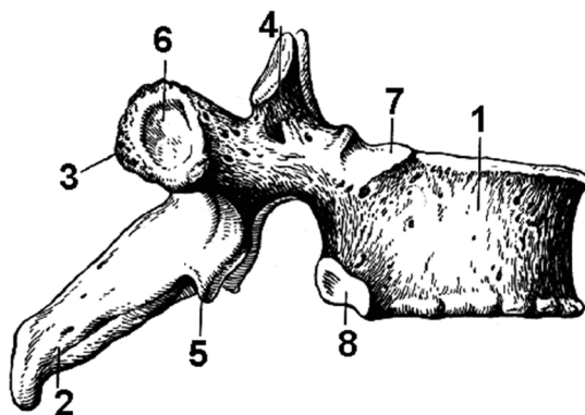
Рисунок 2 – Позвонок человека.
