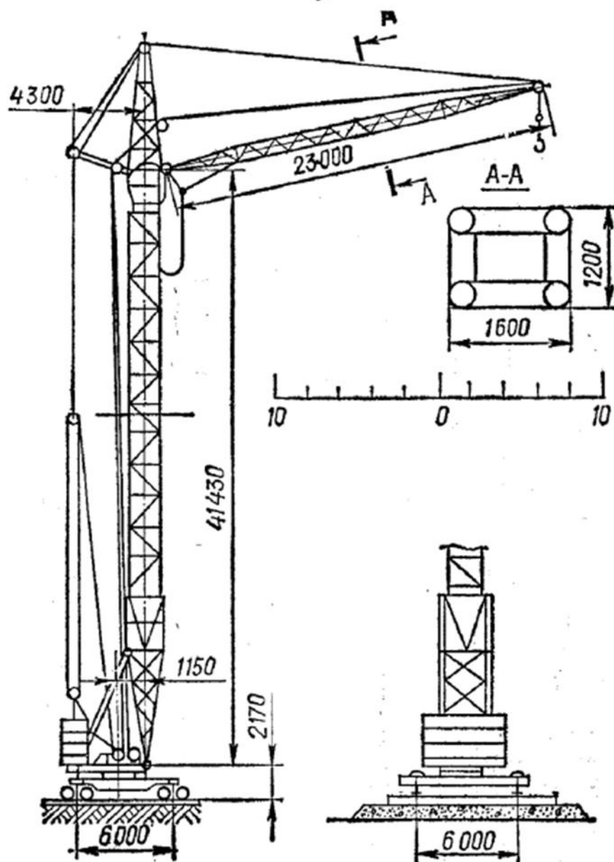
Рисунок 18– Схема крана КБ-160.2
