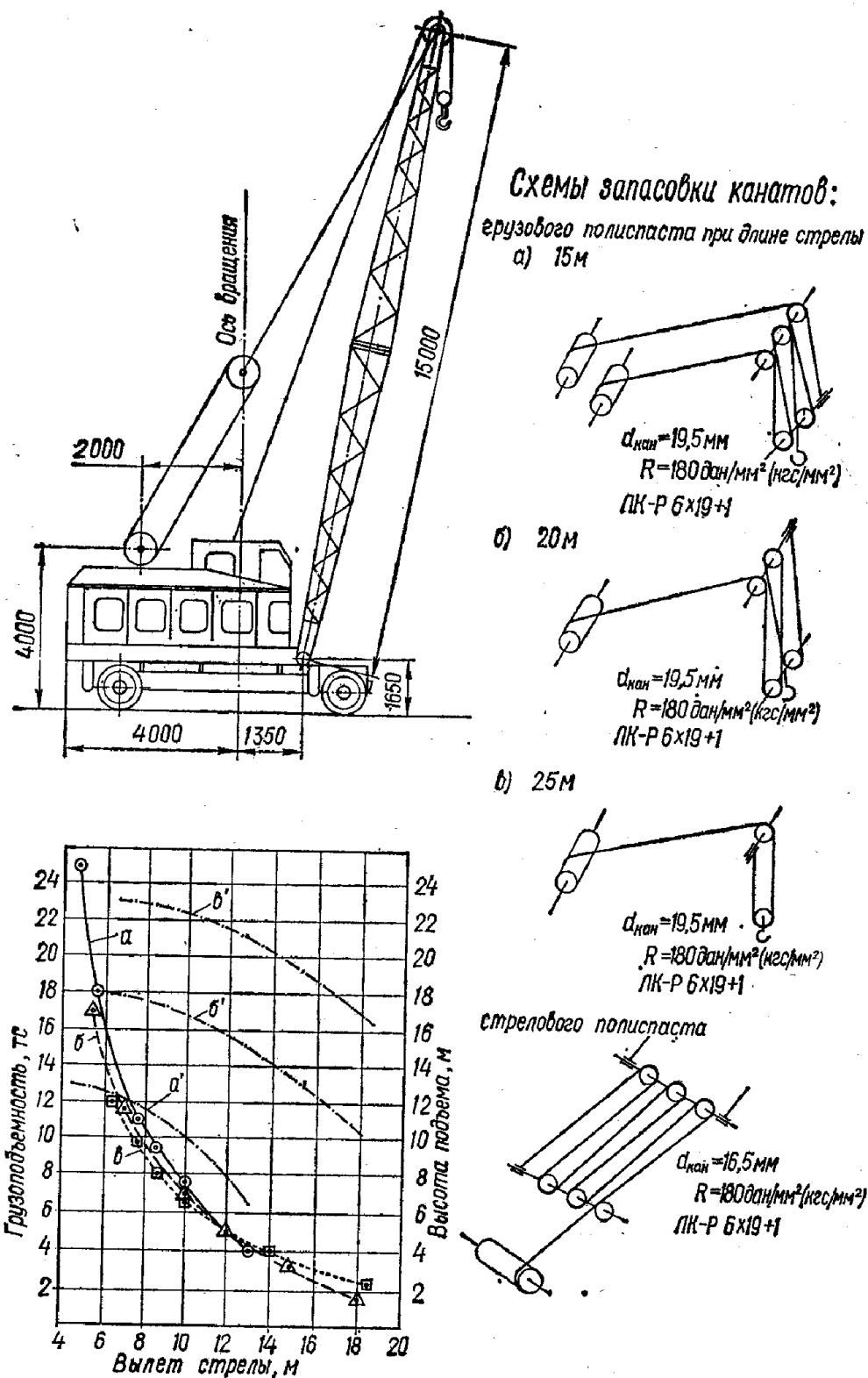
Рисунок 26 - схема пневмоколесного крана КС-5361, график его грузоподъемности и схемы запасовки канатов при различной длине стрелы: d_{кан} - диаметр каната; R - временное сопротивление разрыву отдельной проволоки каната; ЛР-Р6х19+1 - формула каната; \alpha , \beta , \gamma - грузоподъемность крана при длине стрелы 15, 20 и 25 м; \alpha' , \beta' , \gamma' - высота подъема крюка при тех же длинах стрелы
