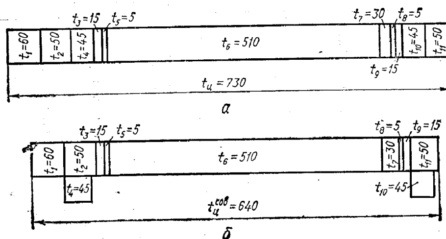
Рисунок 9 - Примерные схемы построения рабочего цикла крана: а – без совмещенных операций; б – при совмещении операций
