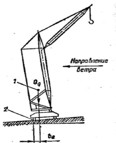
Рис. 14. К определению собственной устойчивости крана: 1 — центр тяжести крана; 2 — ребро опрокидывания.
