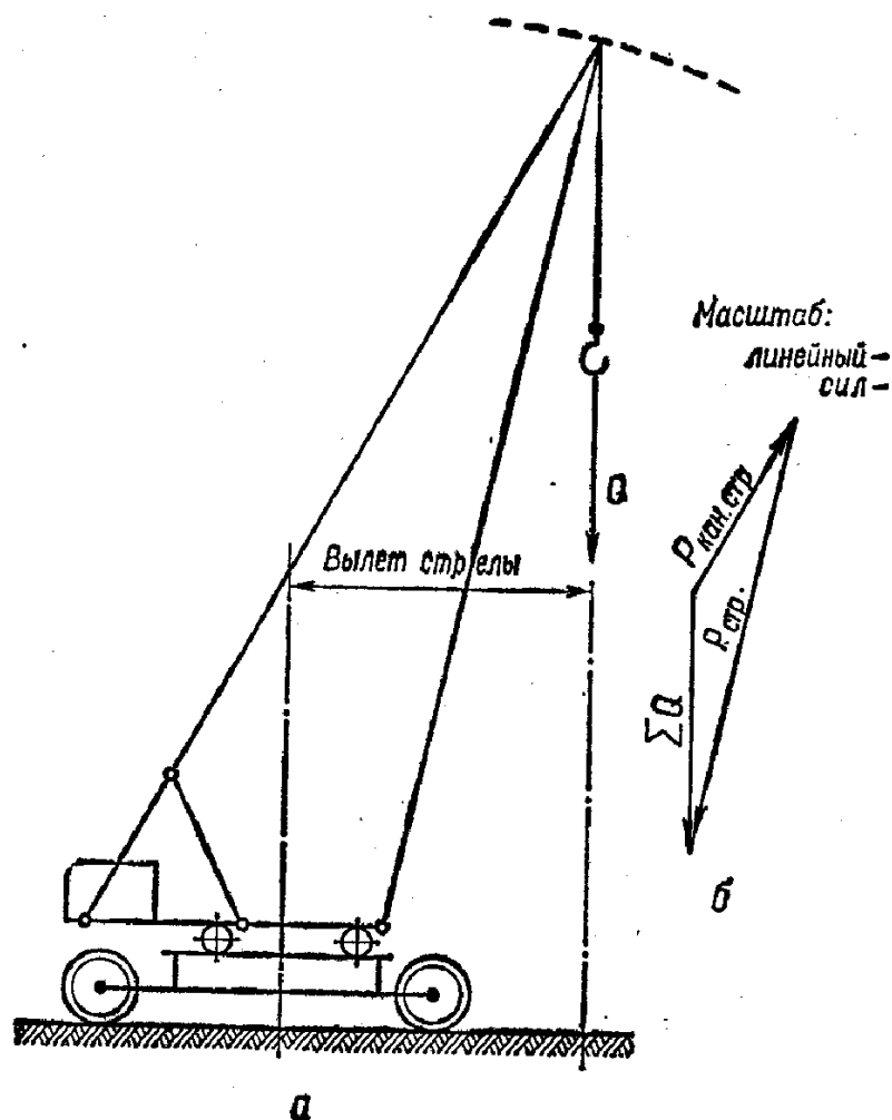
Рисунок 25- Пневмоколесный кран: а- расчетная схема; б- силовой треугольник
