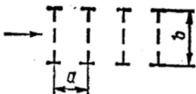
Рисунок 21- Схема расположения ферм или сплошных балок к определению аэродинамического коэффициента
